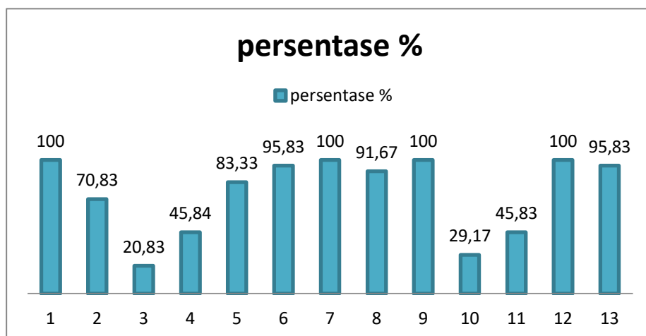
Gambar 2.1 Diagram Batang Kesulitan Siswa Menuliskan Lambang Bilangan
