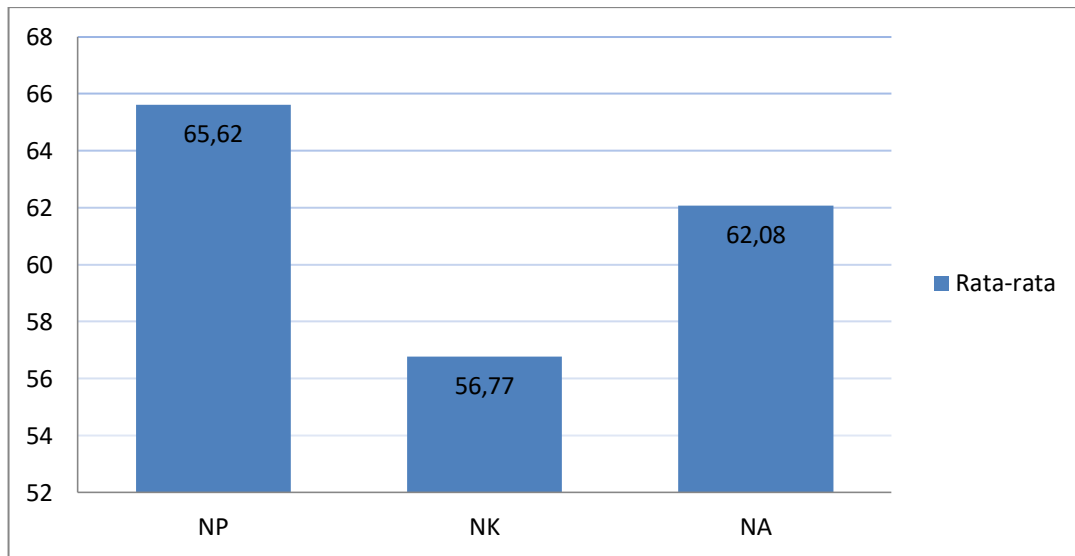
Gambar 1.1 Diagram Batang Kemampuan Siswa Menuliskan Lambang Bilangan.
